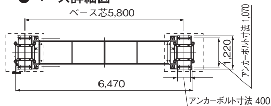
●ベース詳細図
