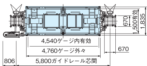
●ベース詳細図
