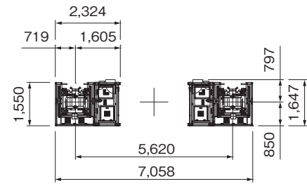
●頂部連台平面図
