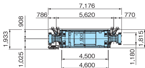
●搬器平面図
