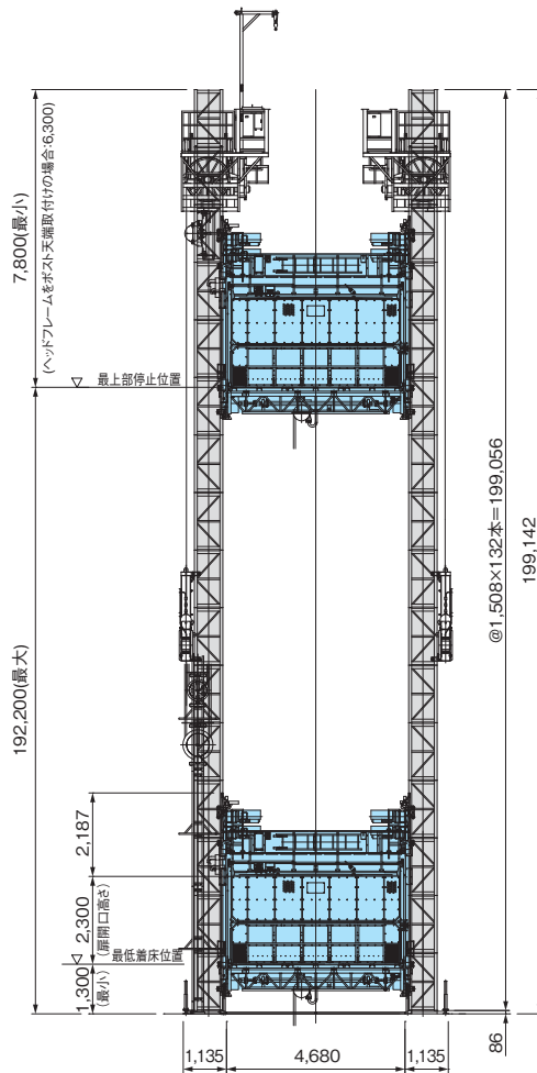
●主要寸法図
