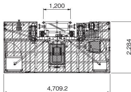
●連台平面図
