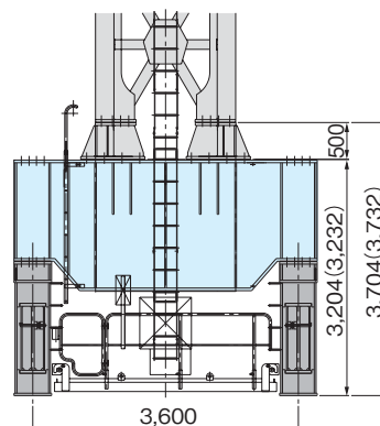
□-1,900マスト取付状態
