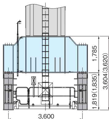
JCC-400H形マスト取付状態
