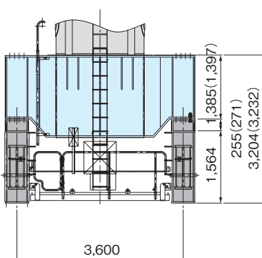
JCC-V720S形マスト取付状態
