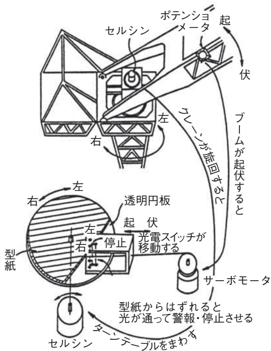
作動原理
