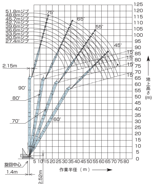
●ラフニングクレーン作業範囲図
